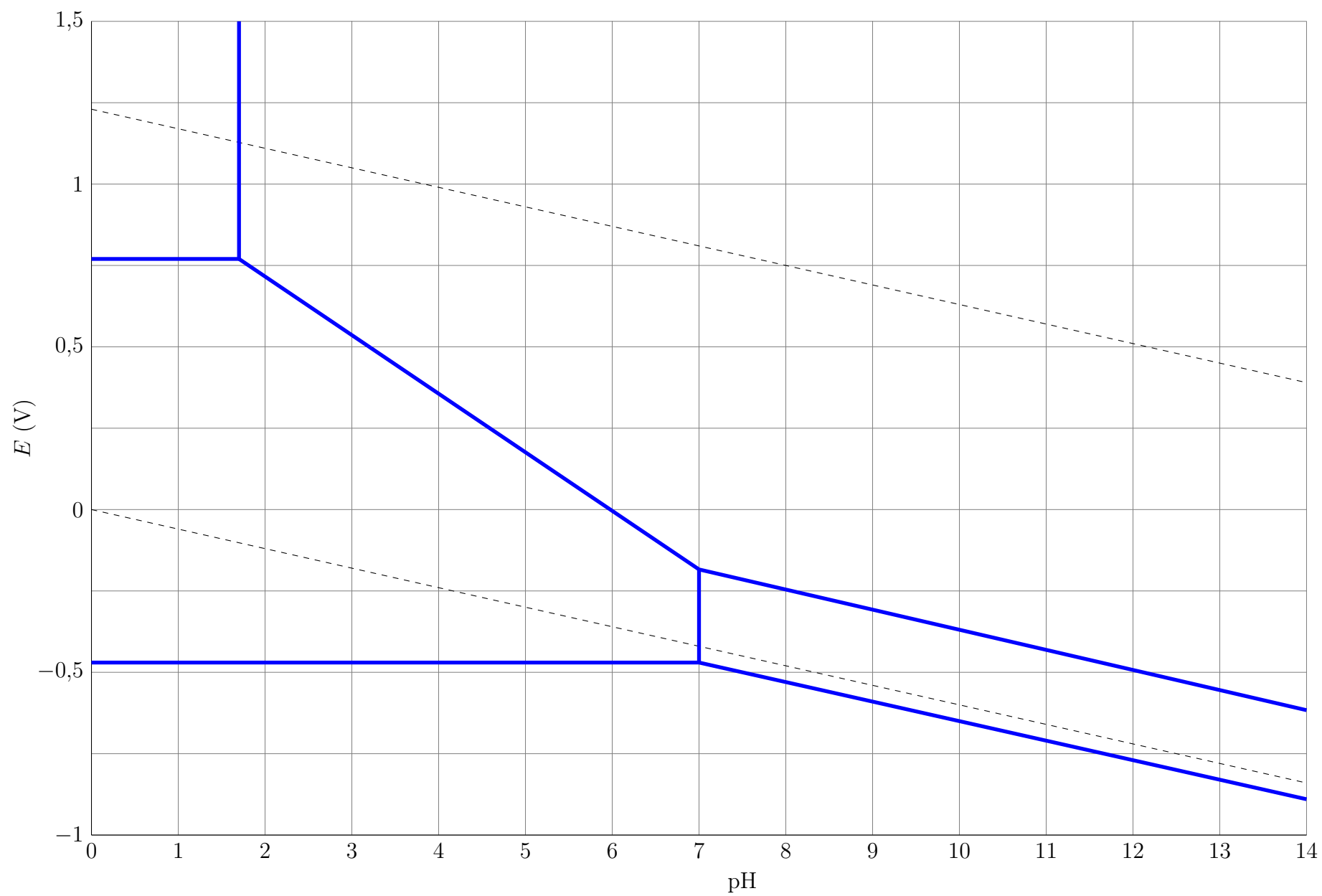
Diagramme E-pH du fer avec une concentration de travail c = 1,0 \times 10^{-1} \text{ mol.L}^{-1}
